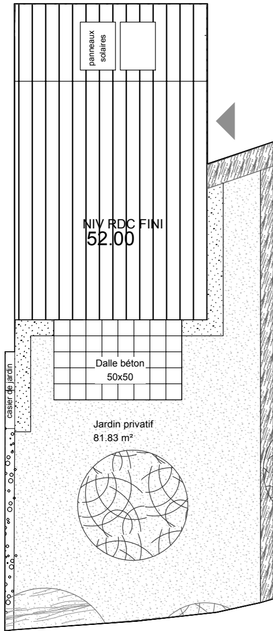
Plan Masse
