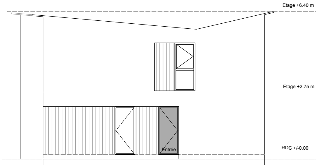
Elévation Est Lot N° 4
